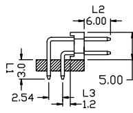
R1 TYPE
