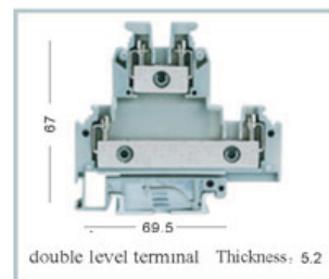
UKKB3
