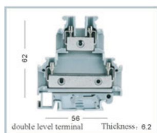
UKK5
