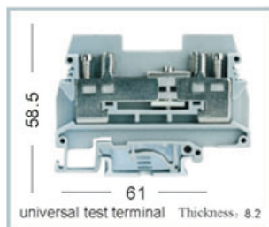
URTK/S
