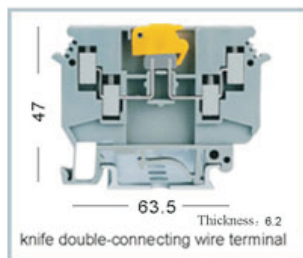
UKD4-P/P
